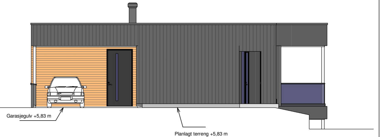
Fasade mot nord 1 : 100
