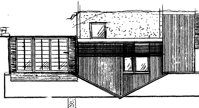
FASADE VEST
