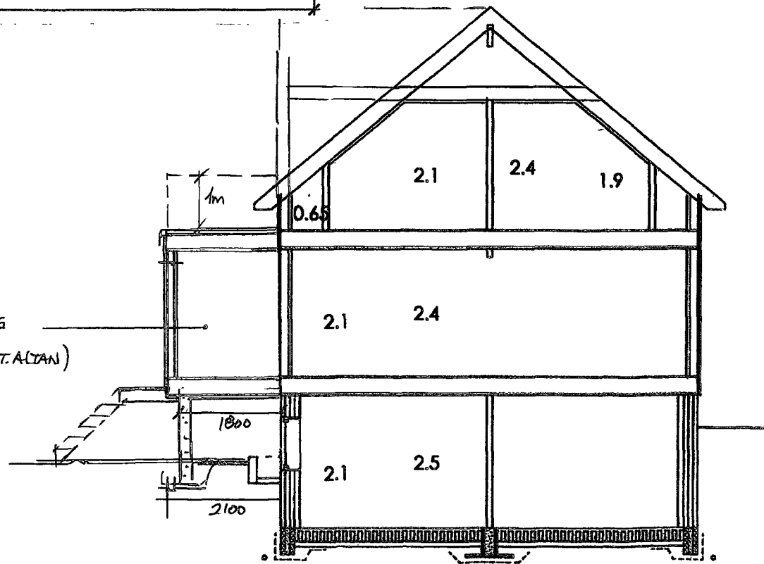
Snitt A-A
