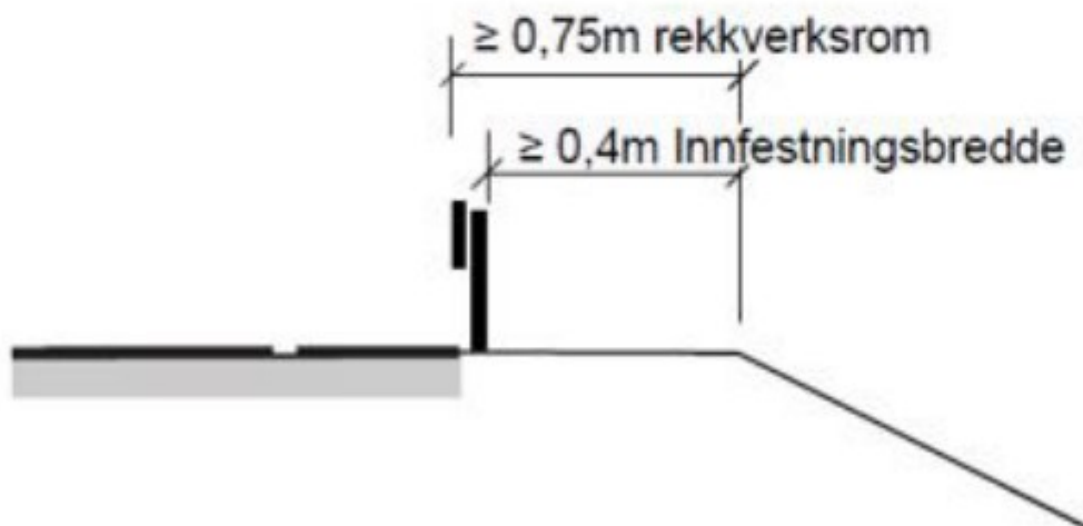
Figur 4.2.2—1 — Krav til plassering av rekkverk i rekkverk
