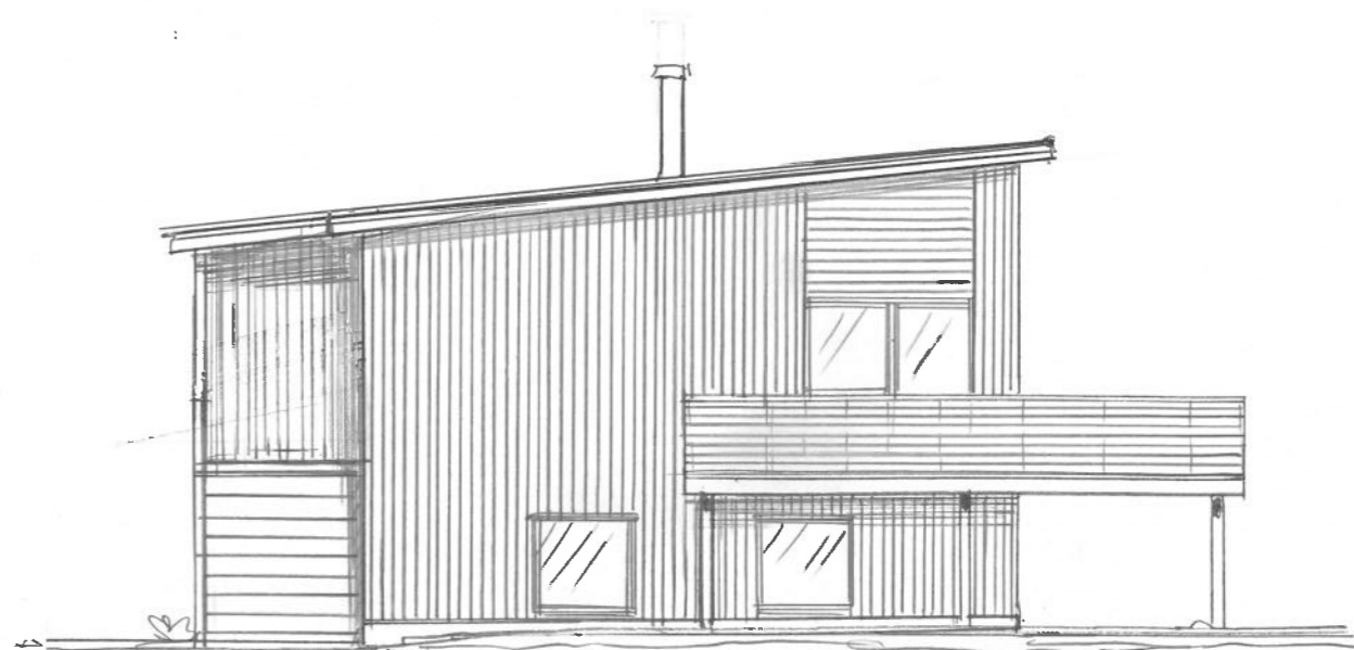
FASADE VEST
