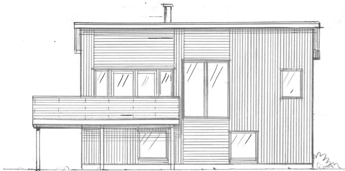
FASADE SØR
