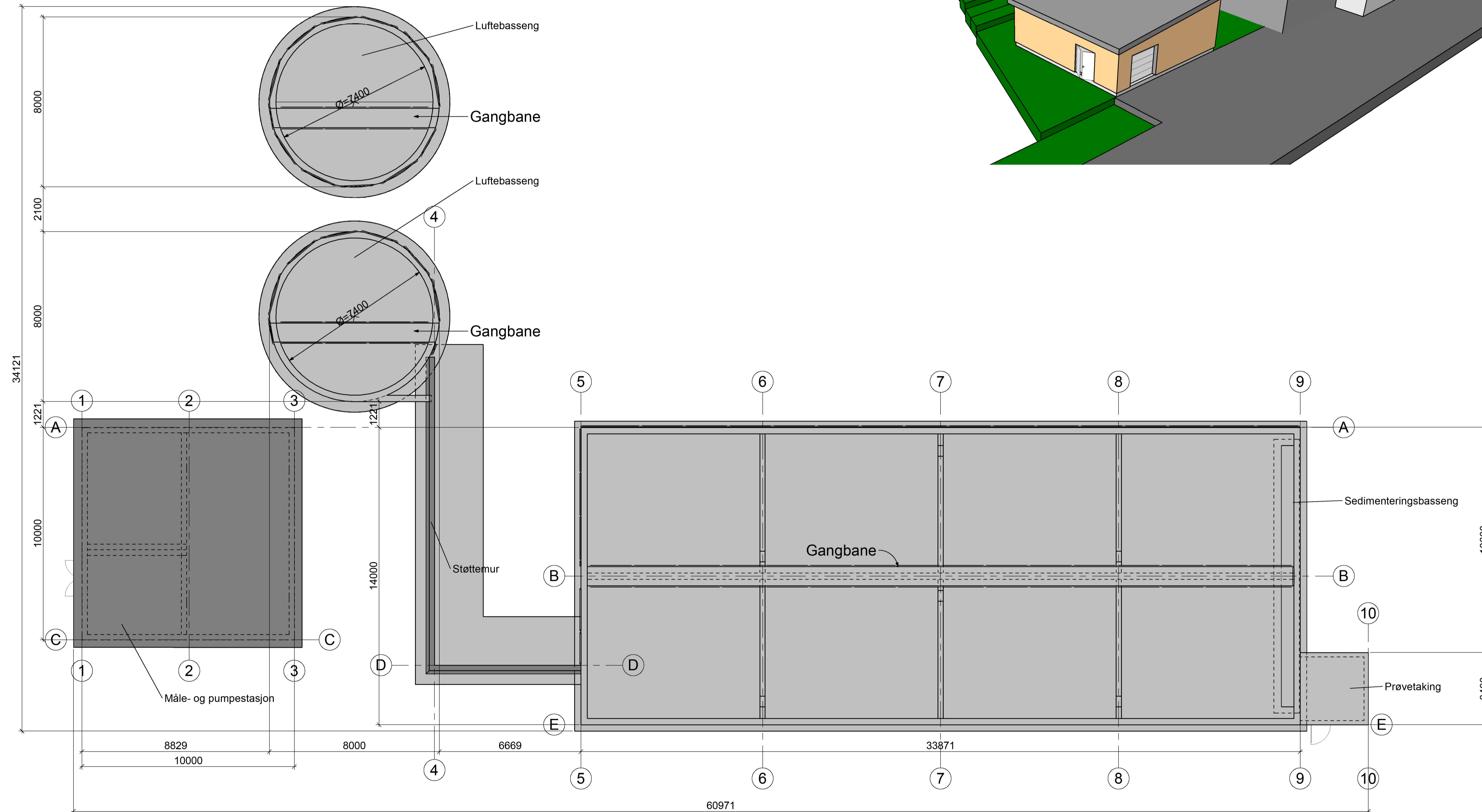
Plan - oversikt 1: 100
