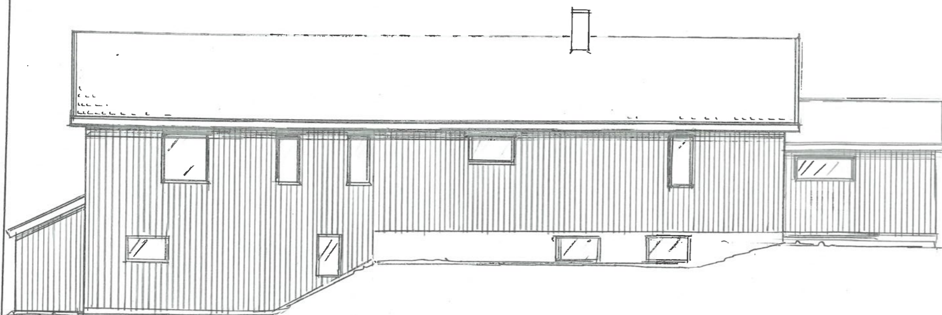
FASADE NORD
