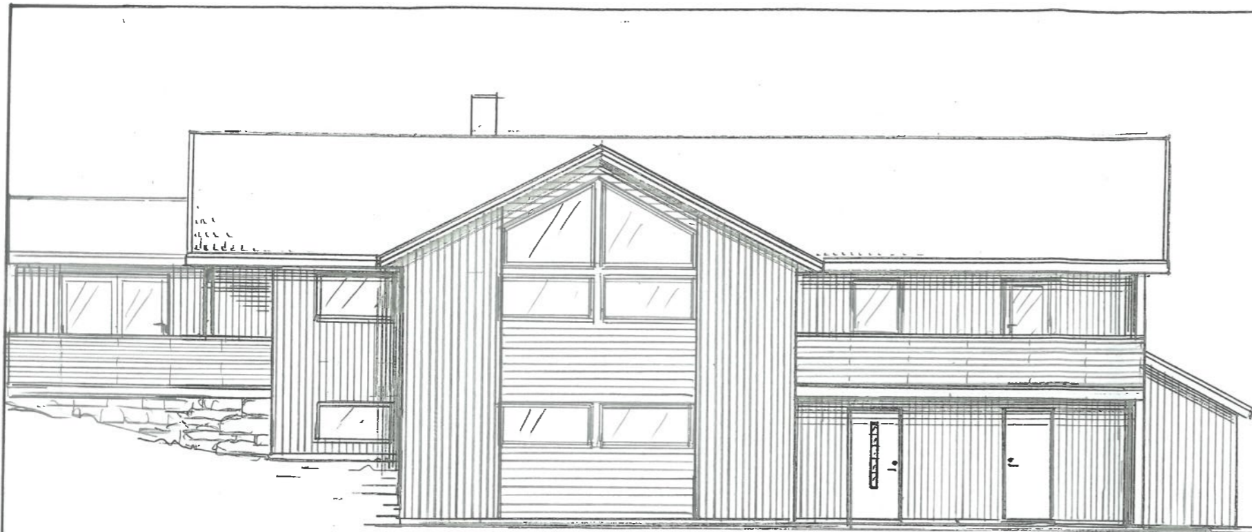
FASADE SØR
