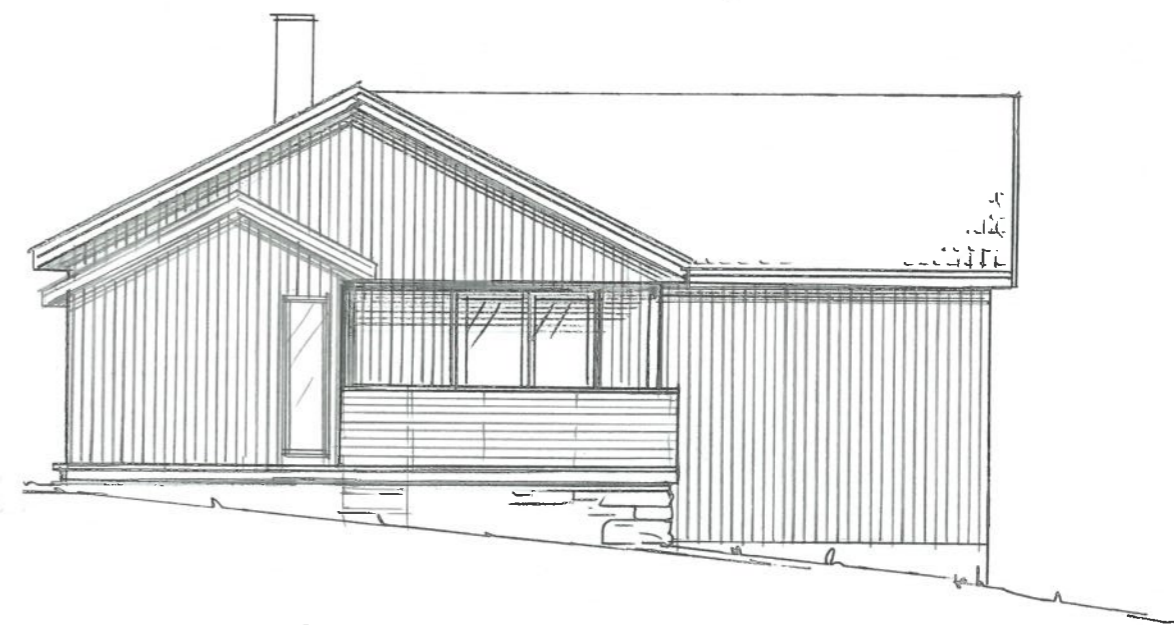
FASADE VEST
