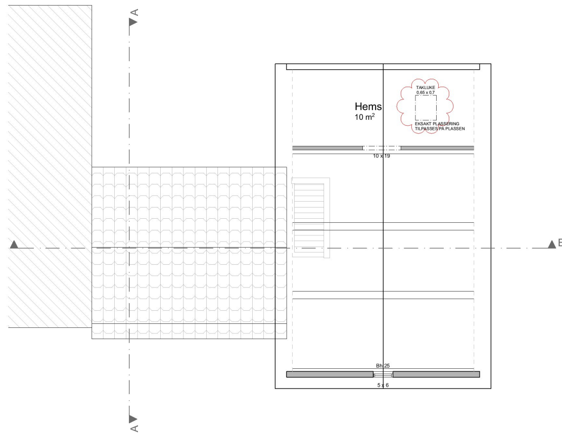
ØVRE DEL 2. ETASJE
