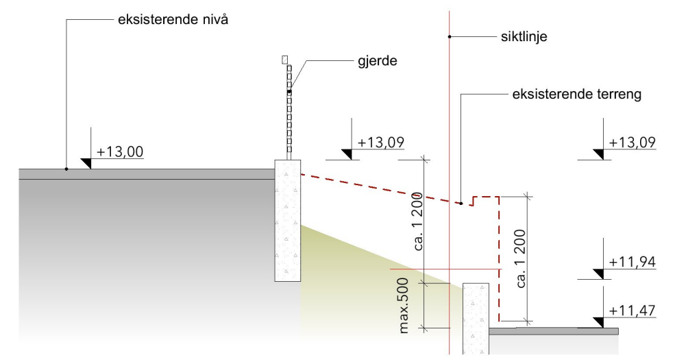
1:50 Snitt S
