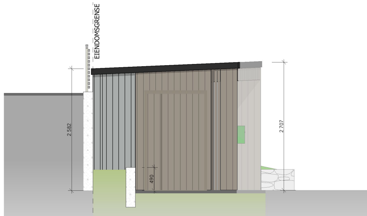
Fasade øst
