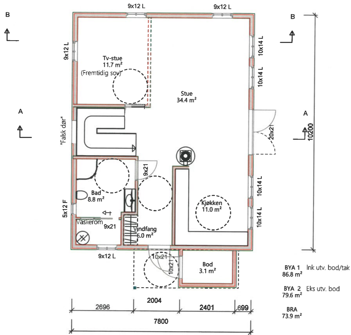
Plan 1.etg
