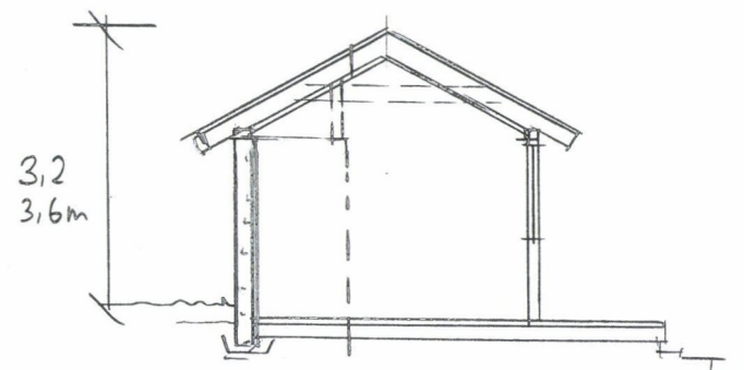
SNITT
