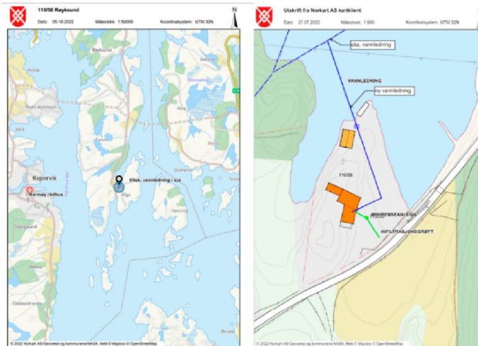
Figur 1: Tiltaksområde for legging av vannledning 2 .
