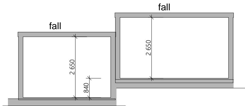
1:100 Snitt A
