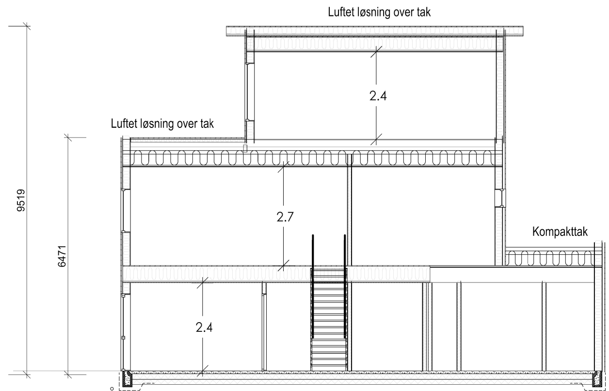
Snitt A:A
