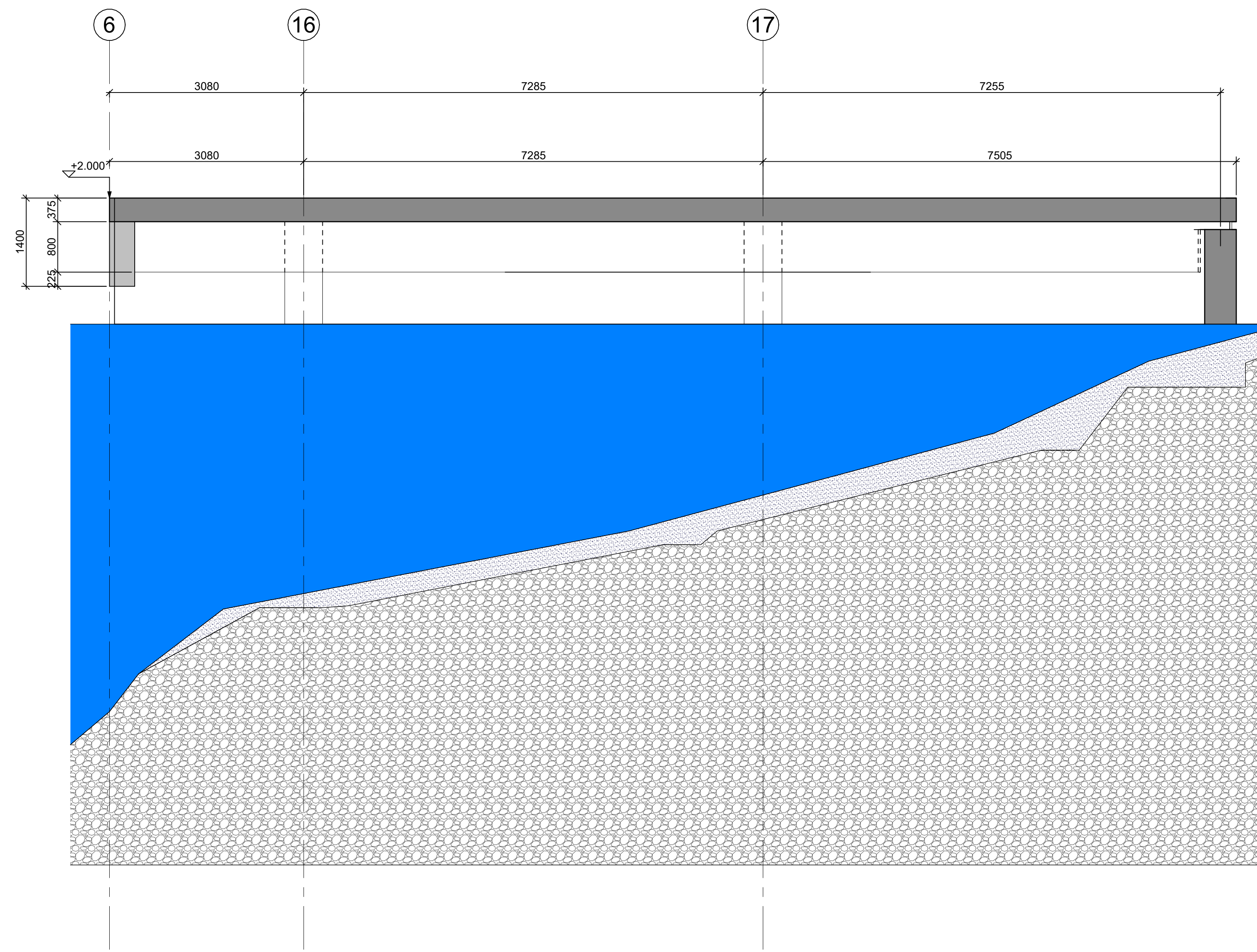
Snitt akse 14 1 : 50
