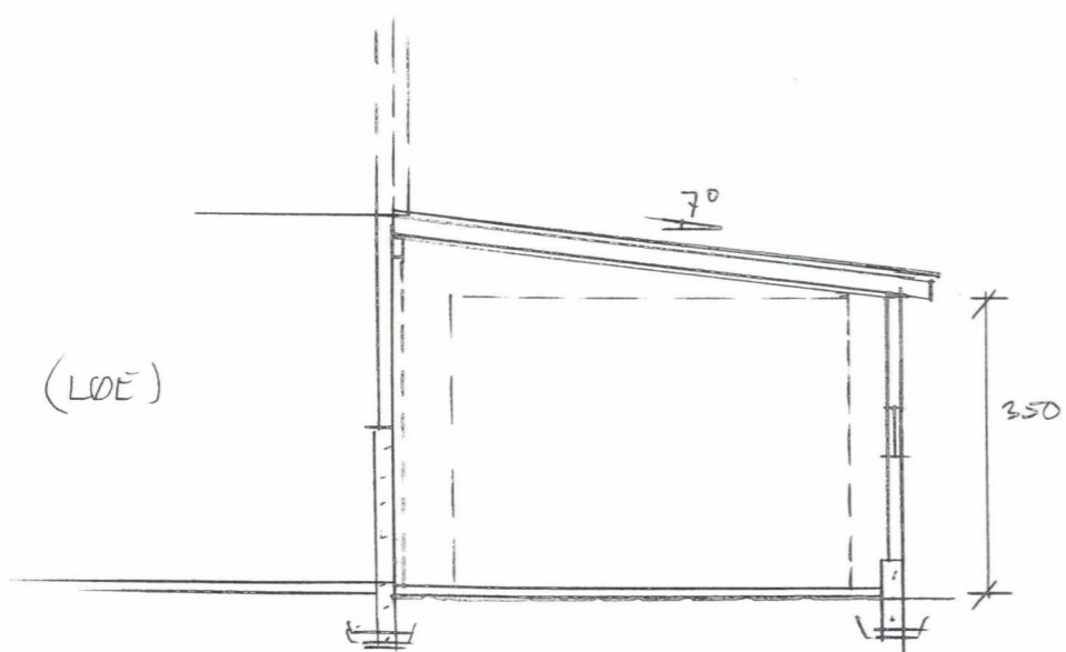
SNITT TILBYGG
