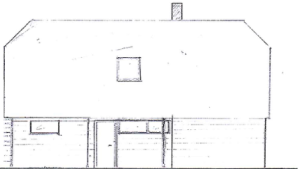
Fasade fra Nord-Vest Etter riving av utestuen Målestokk 1:100
