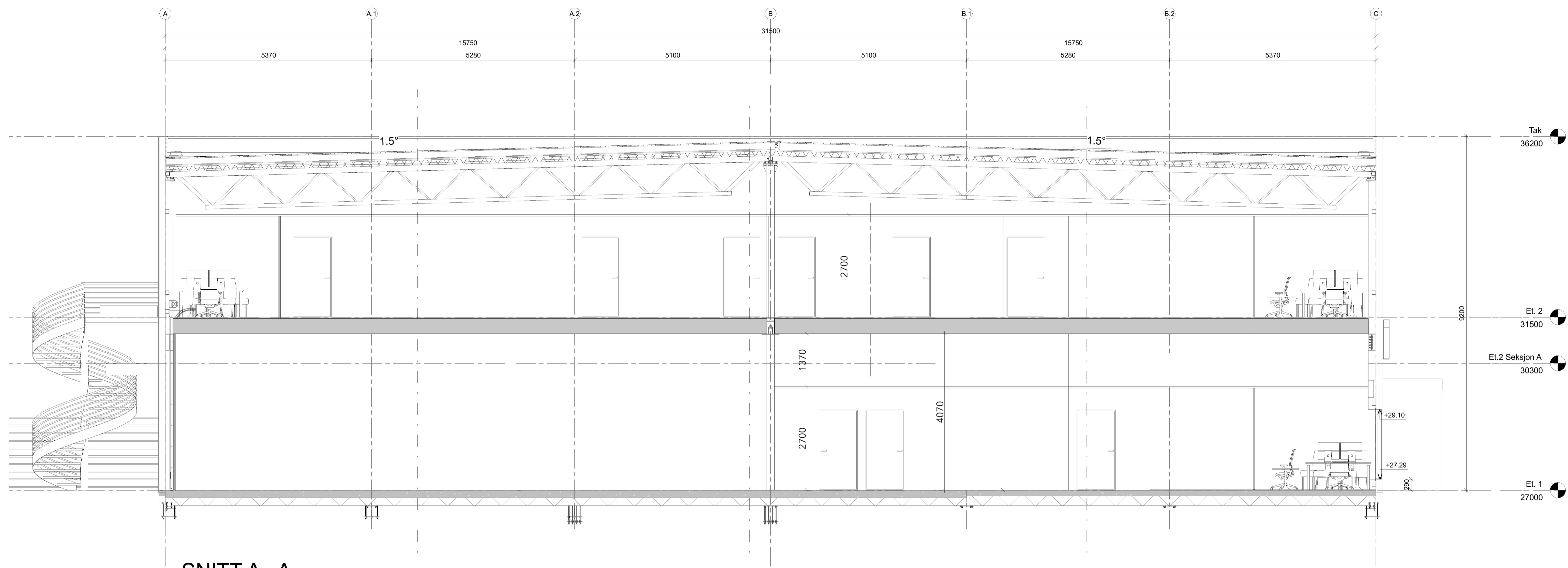
SNITT A - A
