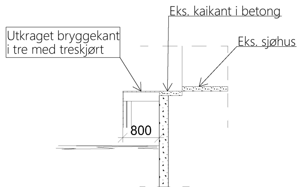
Snitt A-A
