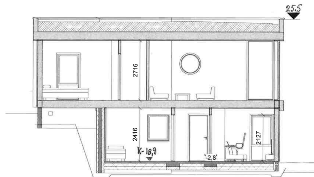
B 1 : 100
