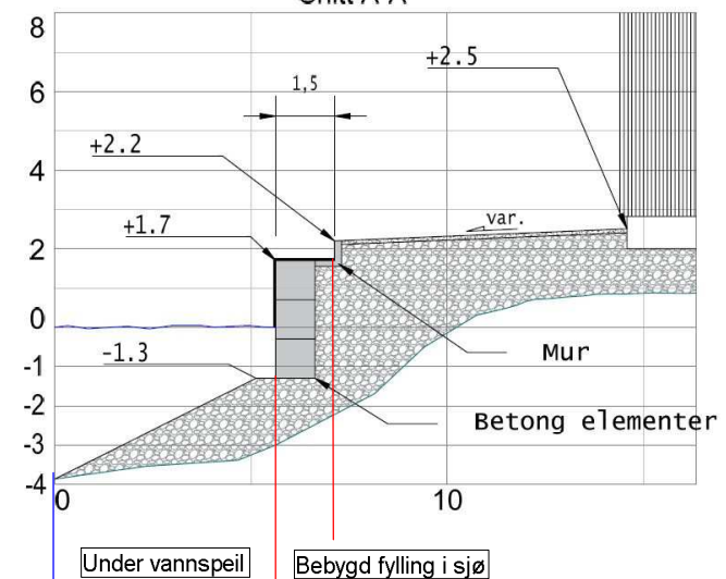
Snitt A-A
