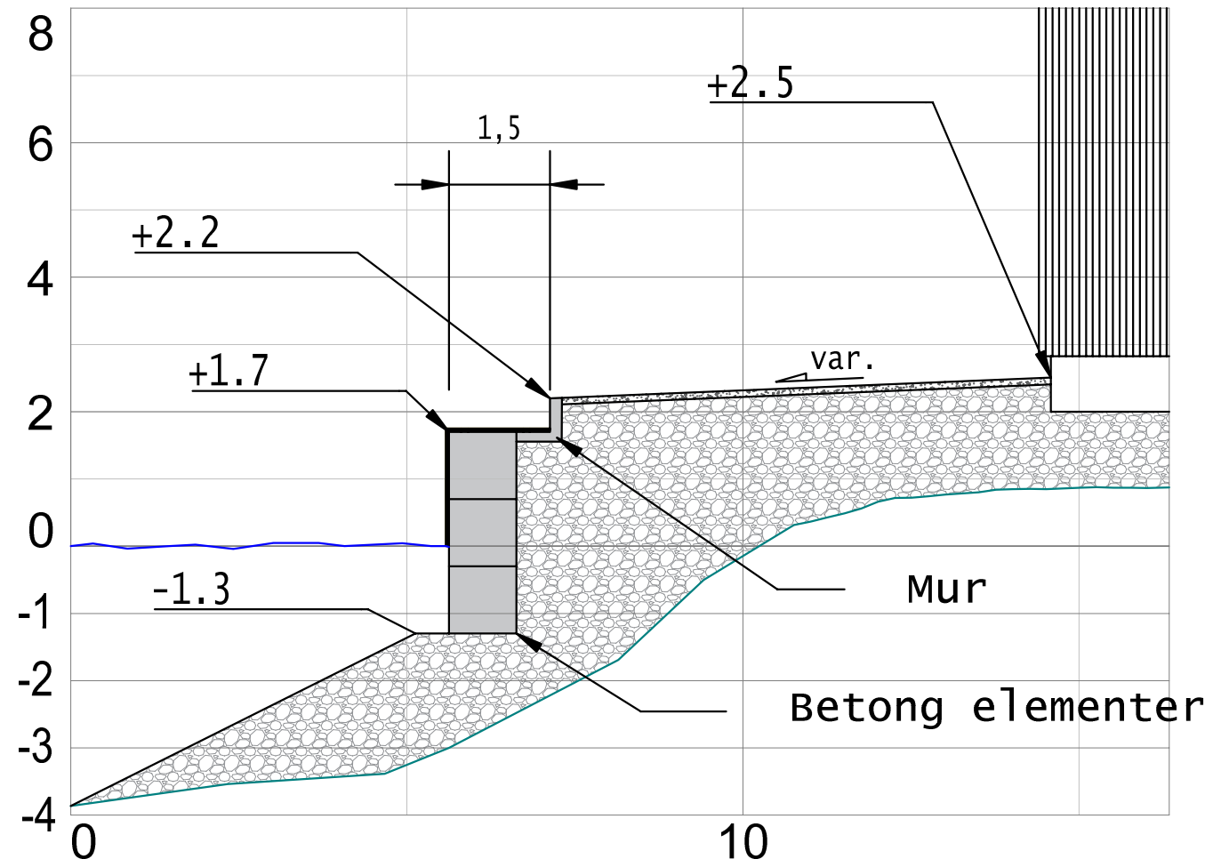
Snitt A-A
