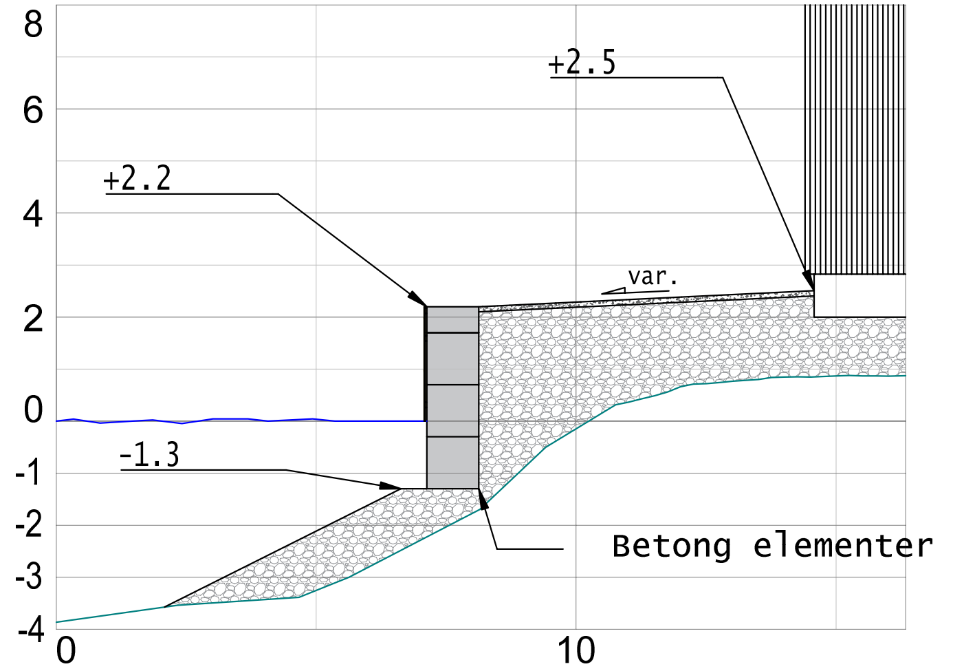
Snitt B-B
