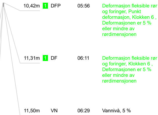
Spillvann_Sluk i dusj 1etg_Påkobling_20201202_104837.jpg
