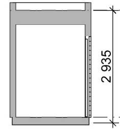
1:100 Snitt A
