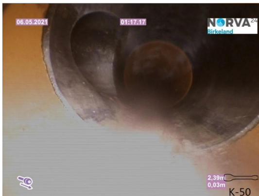
Spillvann_Stakeluke toalett_Påkobling_20210506_122313.jpg
