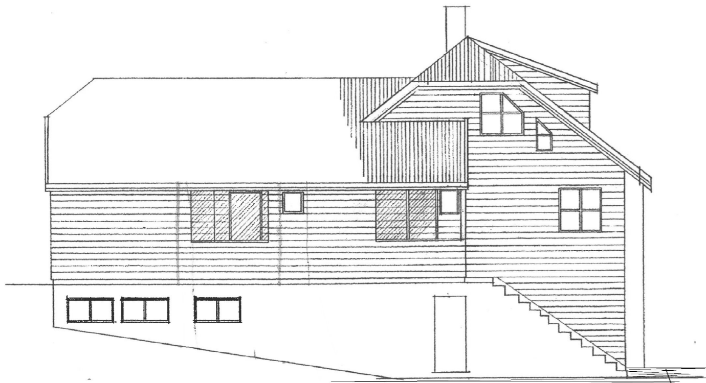
FASADE ØST
