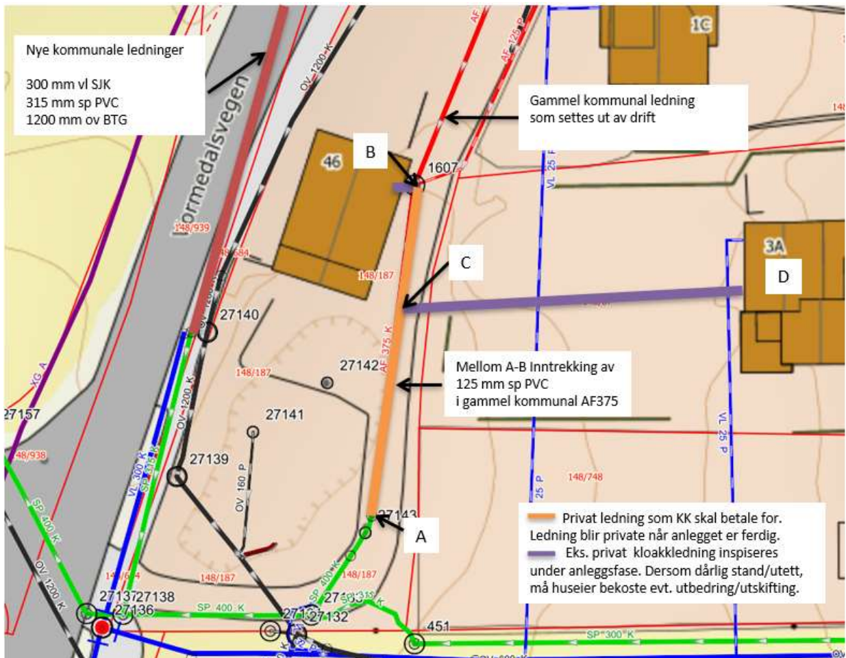
Prosjektert løsning for private stikkledninger Vormedalsvegen 46 og Austbøvegen 3A
