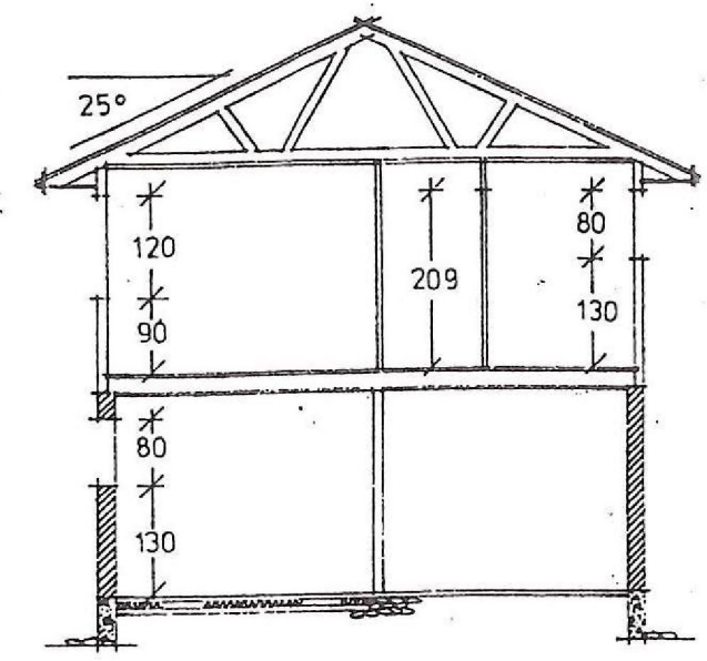
SNITT
