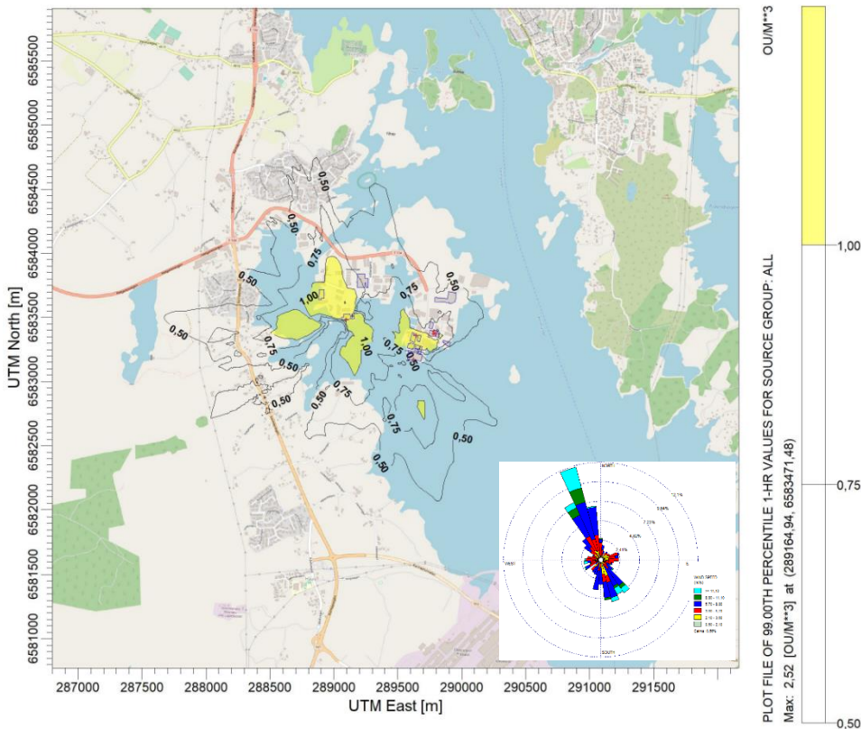
Figur 2: Luktspredningskart for juni måned. Områder som er gule har luktkonsentrasjon over 1 \text{ ou}\epsilon/\text{m}^3 . Ingen boliger ligger i gult område. Vindrosen for juni er vist i nedre høyre hjørne.
