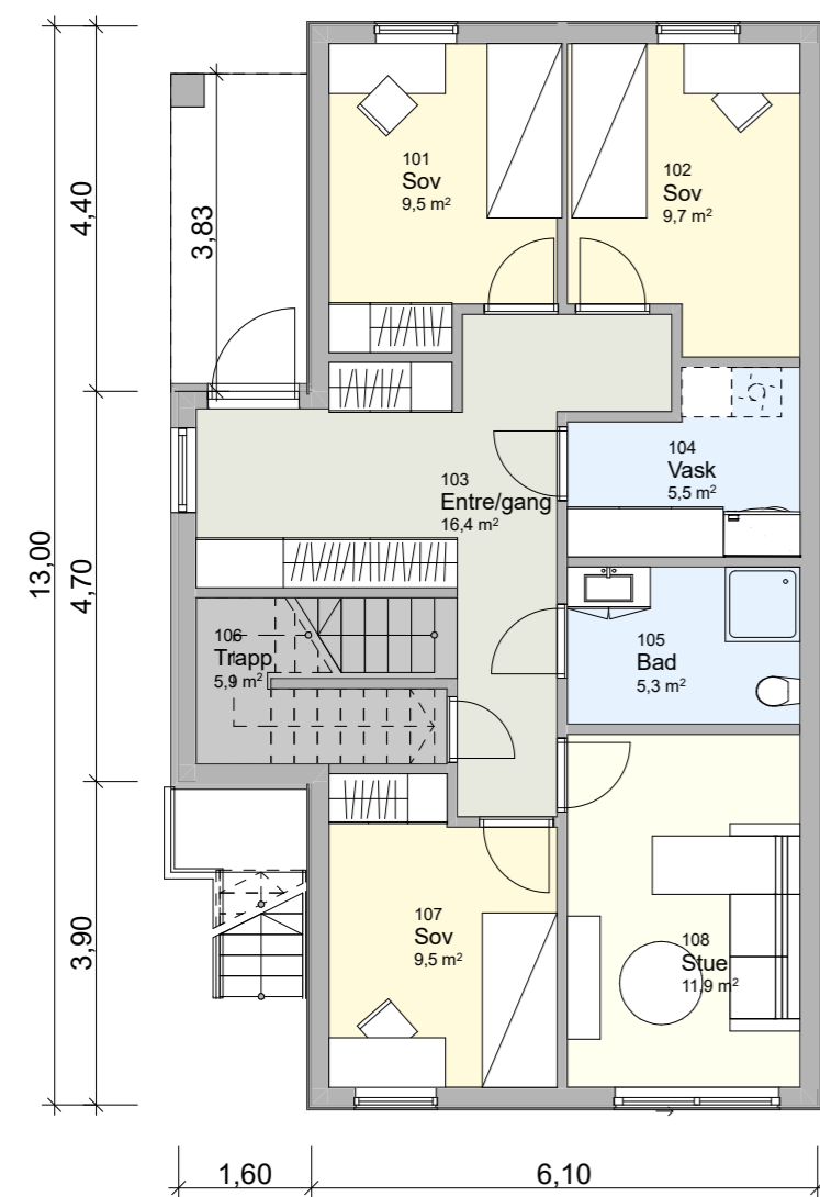
1:100 1. Etasje
