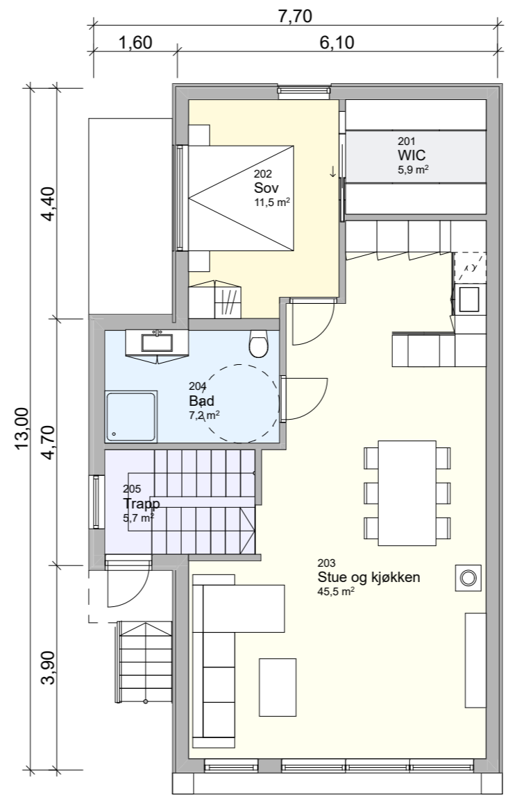
1:100 2. Etasje
