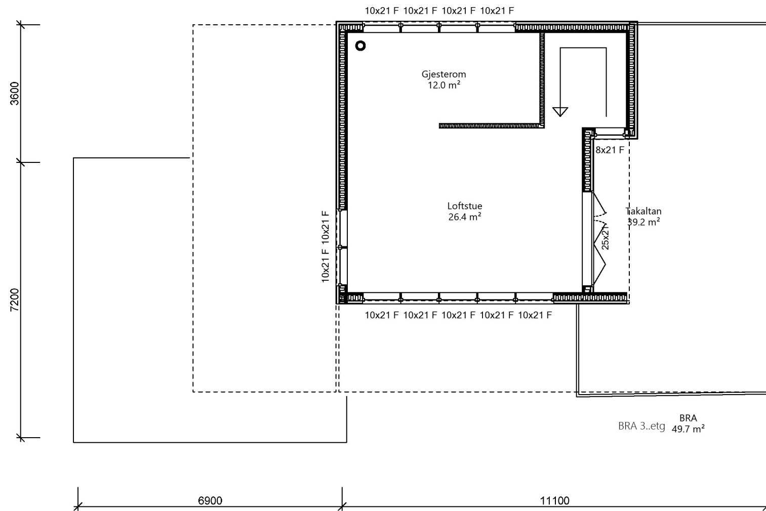
Plan 3.etg
