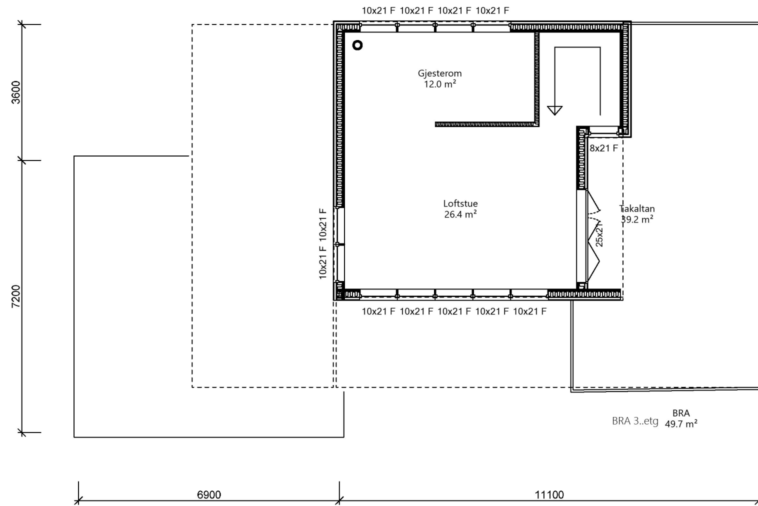
Plan 3.etg
