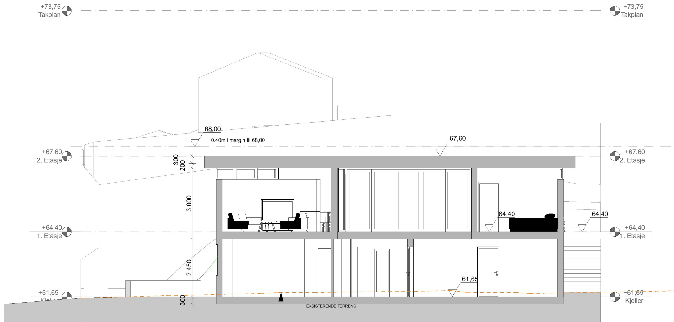
SNITT A-A
