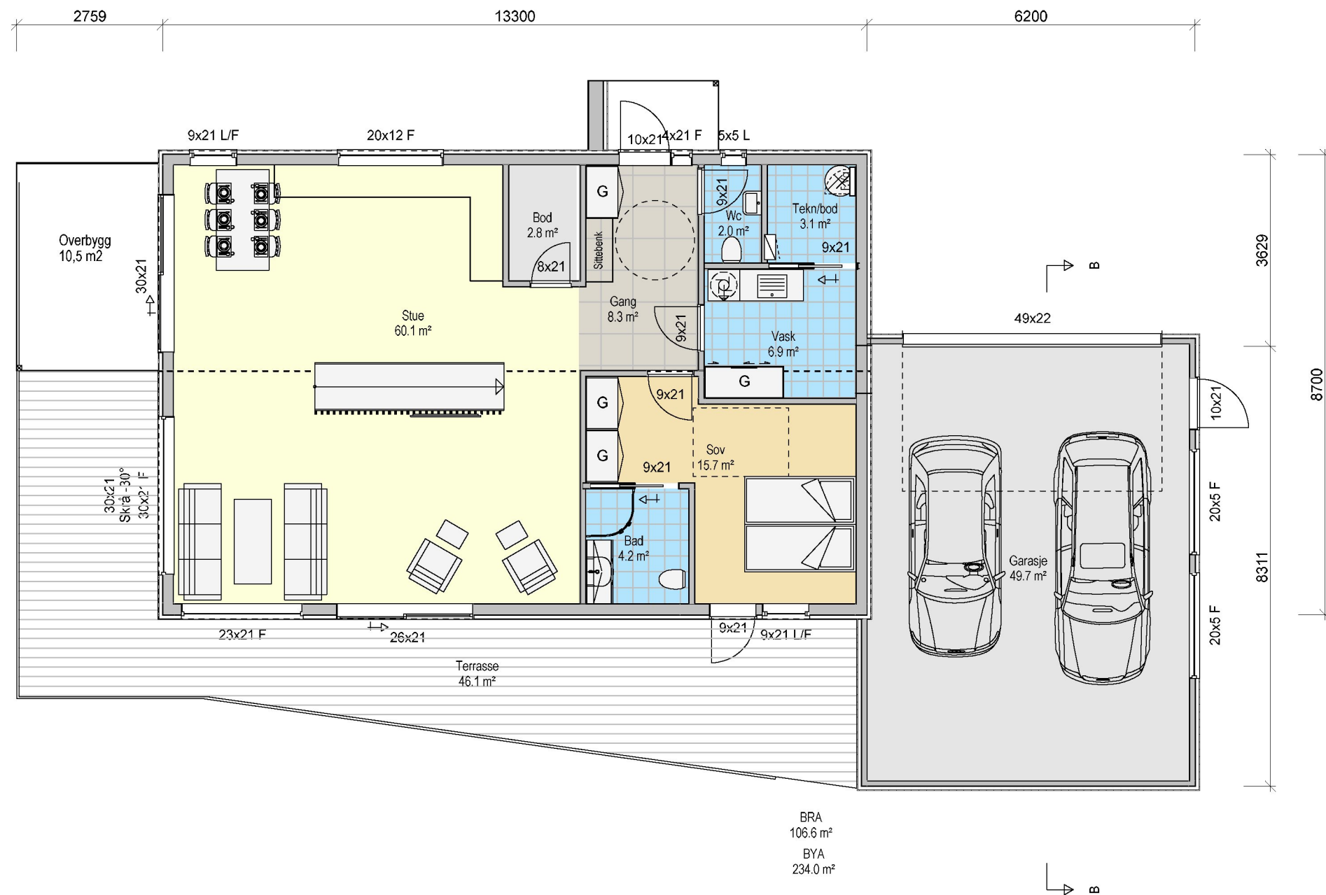
Plan 2 etg
