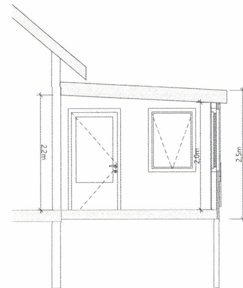
Snitt 1:50
