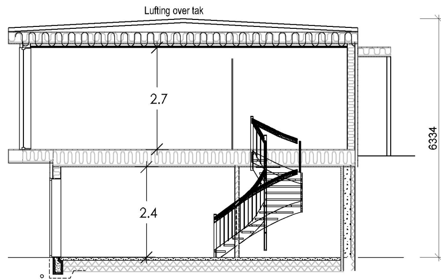
Snitt A:A
