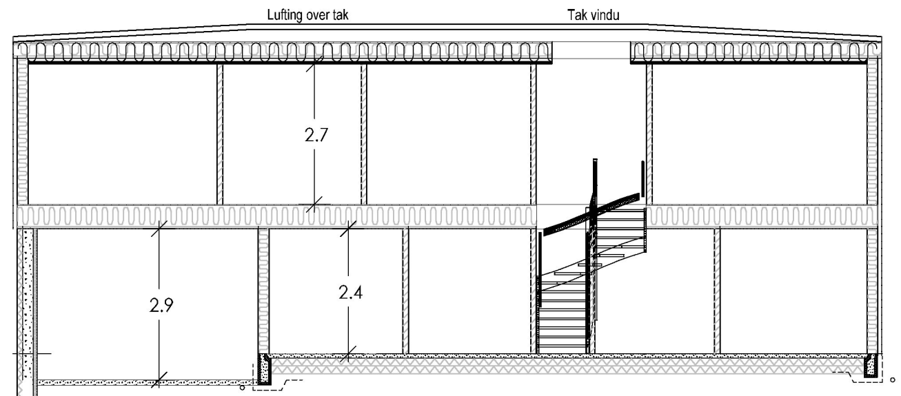
Snitt B:B
