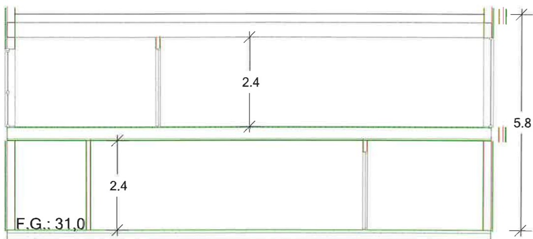
Snitt A-A
