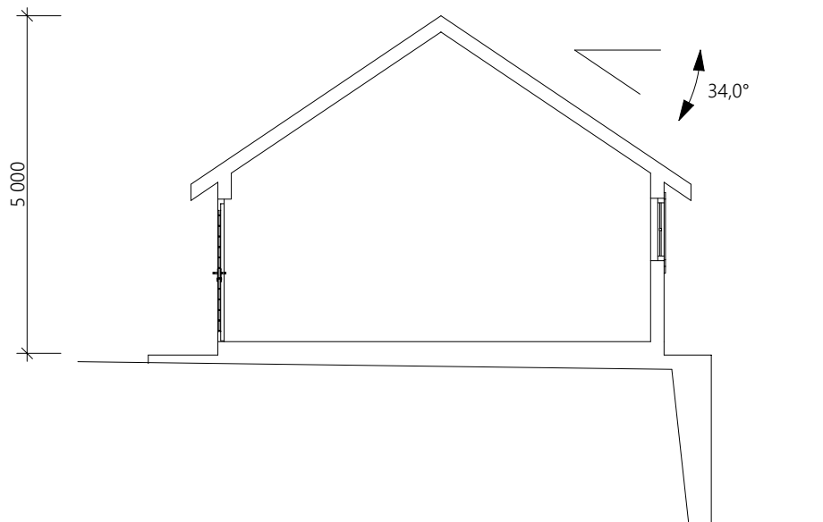
Snitt B
