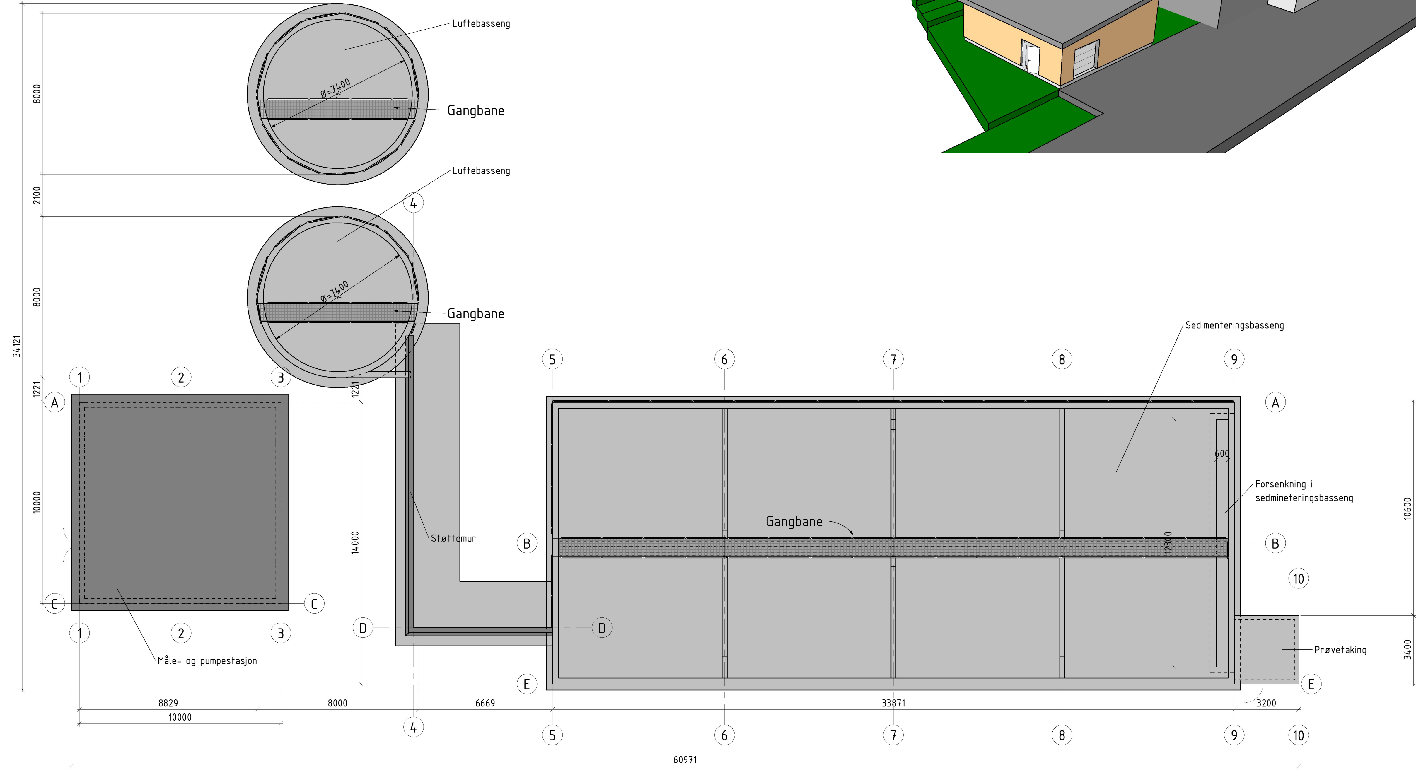
Plan - oversikt 1 : 100
