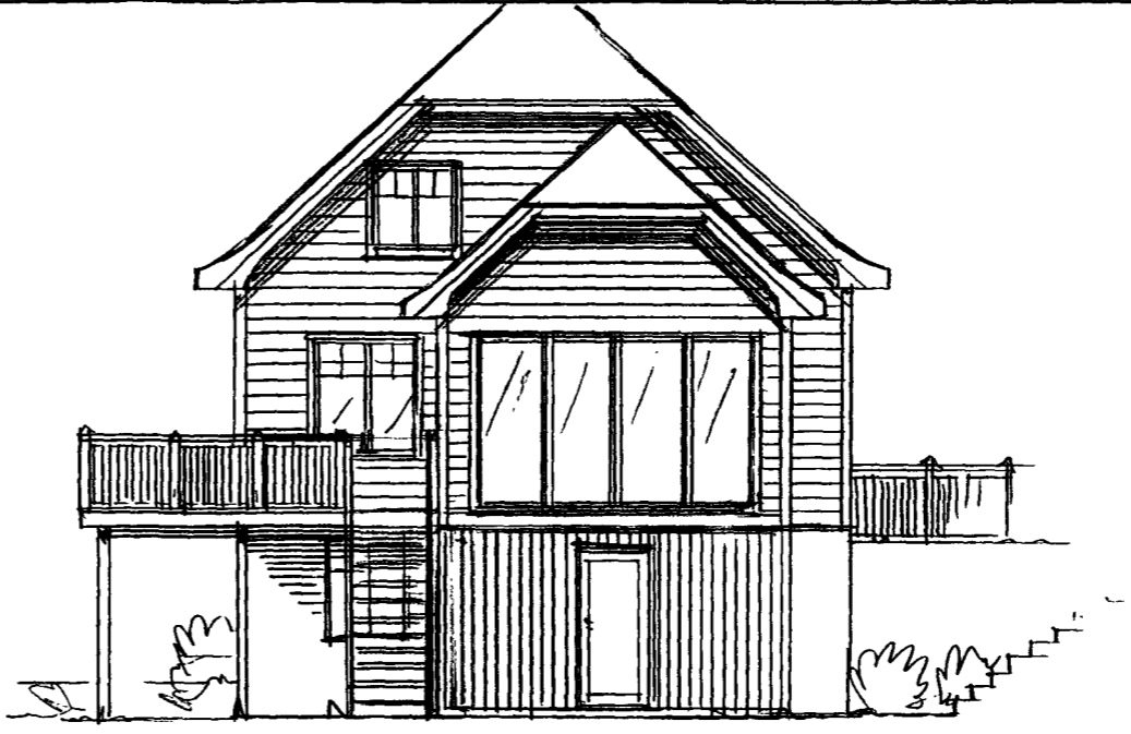
FASADE SØR
