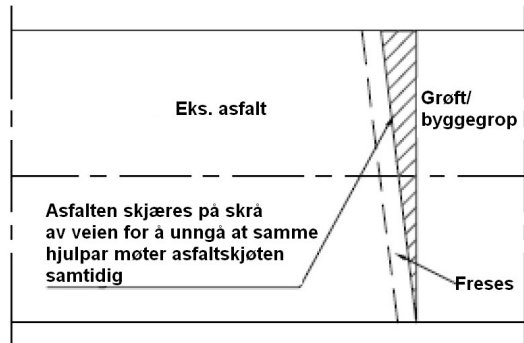
Prinsipp for tilkoping mot eks. veioverbygning- I lengderetning, snitt
