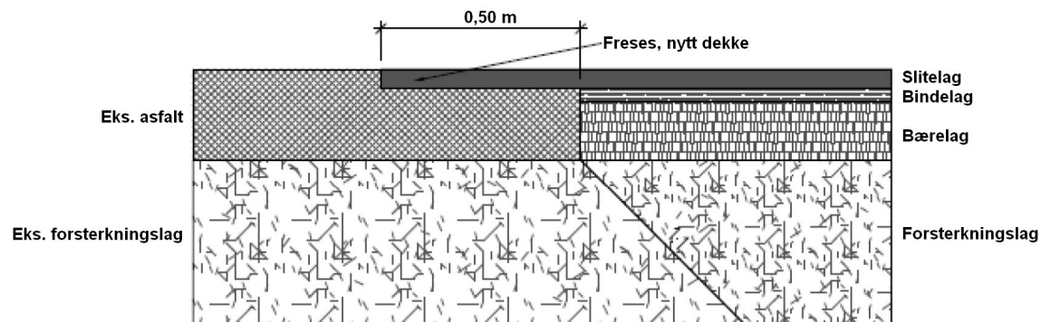
Prinsipp for tilkoping mot eks. veioverbygning - I tverretning, snitt
