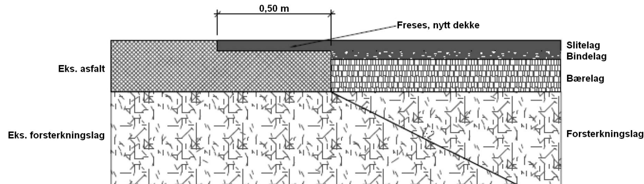
Prinsipp for tilkoping mot eks. veioverbygning- I lengderetning, snitt
