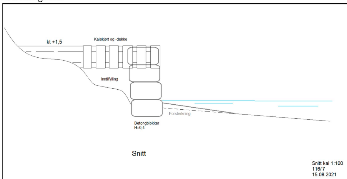
Figur 1: Snitt av planlagt tiltak. Område markert med "forsterkning" skal utfyllast.
