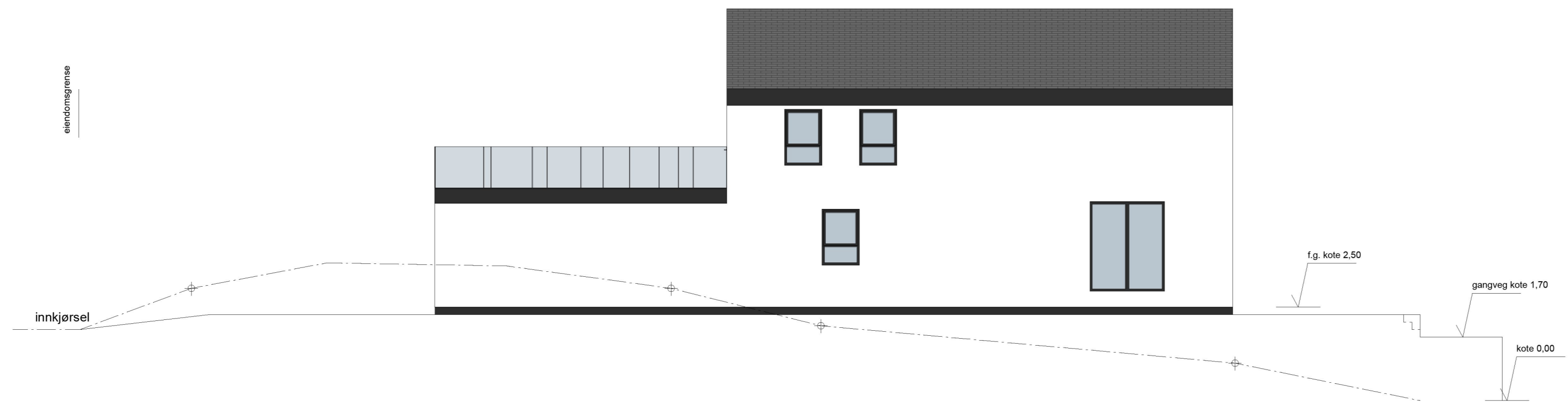
1:100 Fasade Øst
