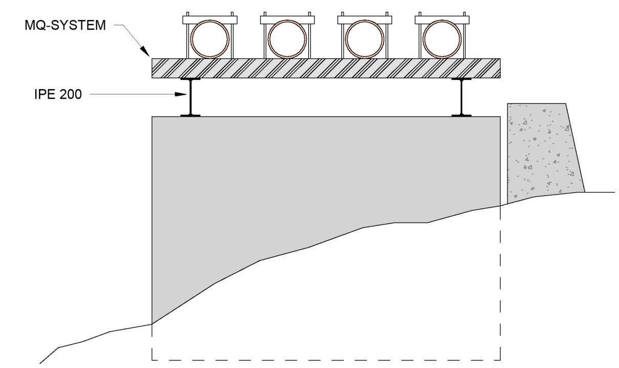
SNITT 1-1 - FORSLAG TIL SUPPORT FOR RØRGATE I DAGEN 1:20
