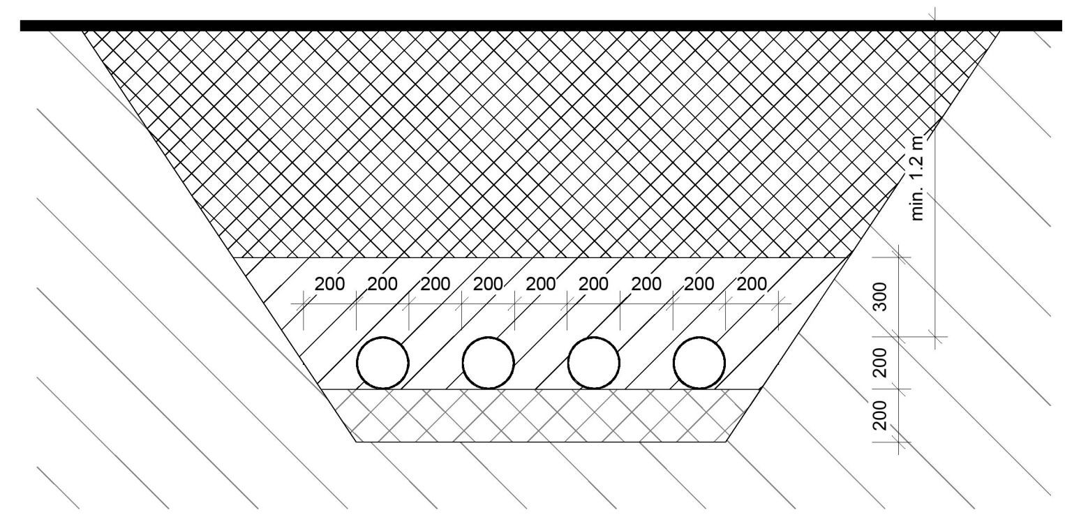
SNITT 2-2 - GRØFTETVERRSNITT 1:20
