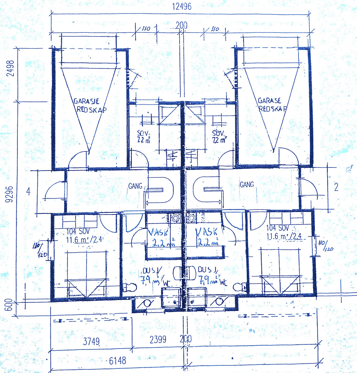
Plan 1. etasje
