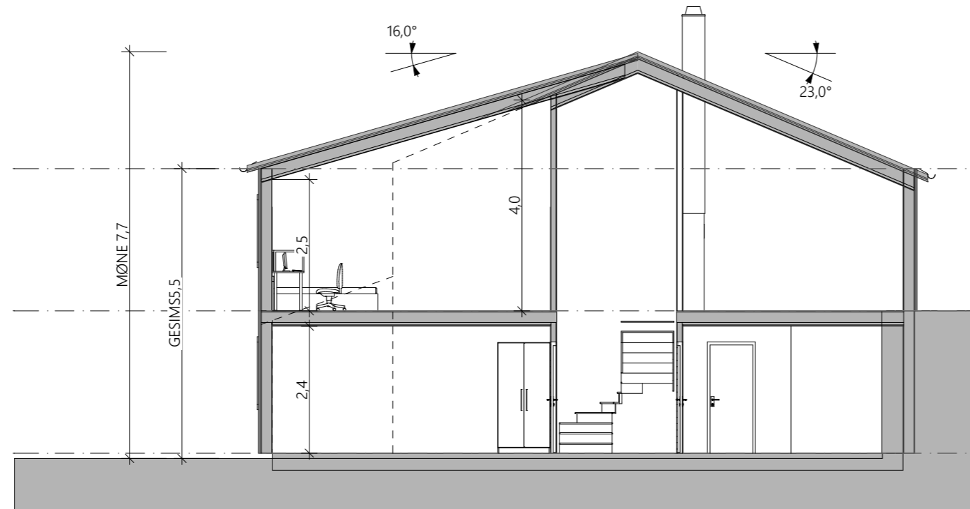
1:100 Snitt A
