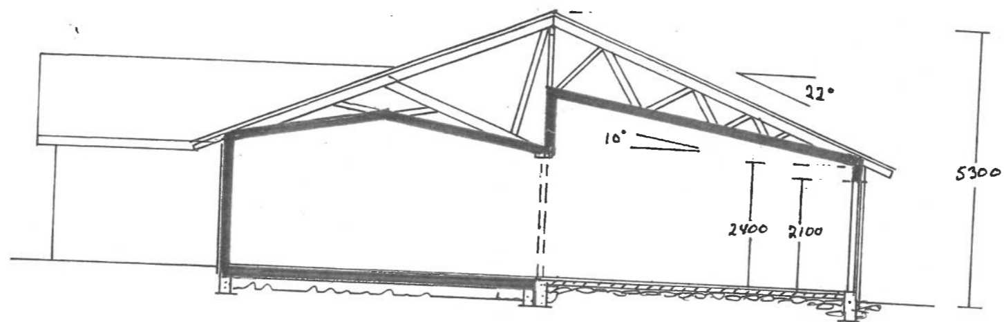
SNITT A-A
