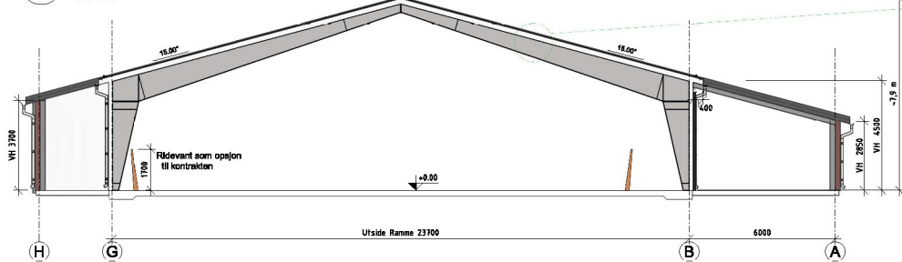
2 Seksjon 1 1 : 100
