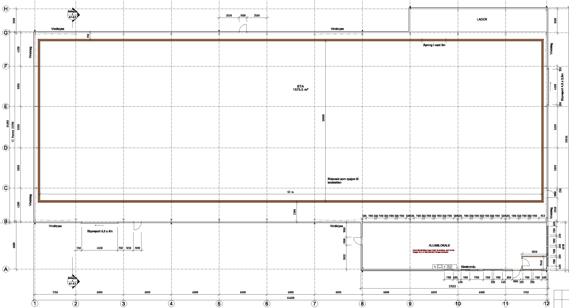
1 Plan 1 1 : 100
