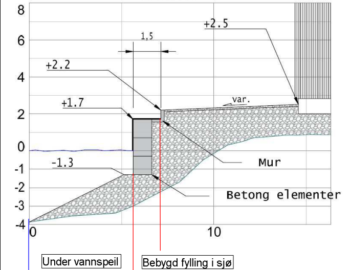
Snitt A-A
